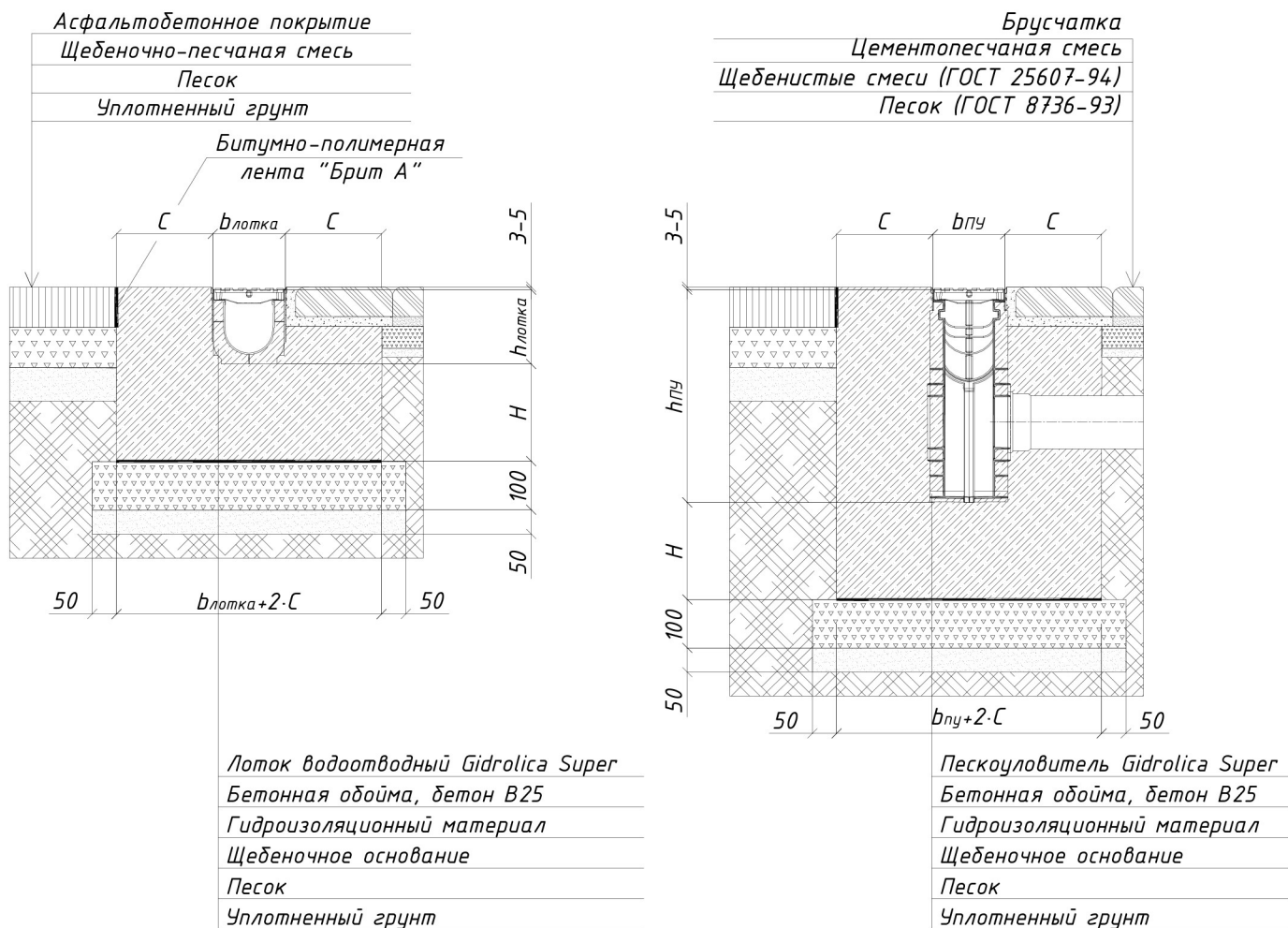
Рис. 1 Схема установки лотка/пескоуловителя у бордюрного камня
